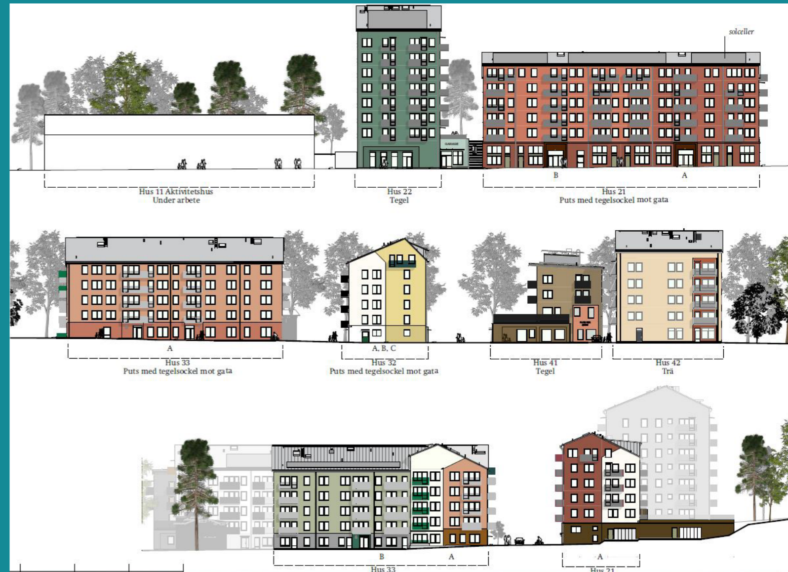
Fasader för föreslagen bebyggelse
