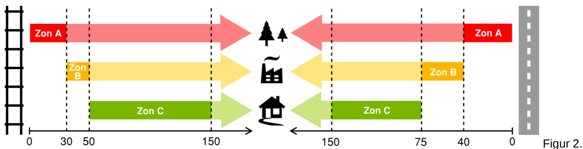
Illustration av rekommendationer till olika typer av bebyggelse utmed väg och järnväg [4].
