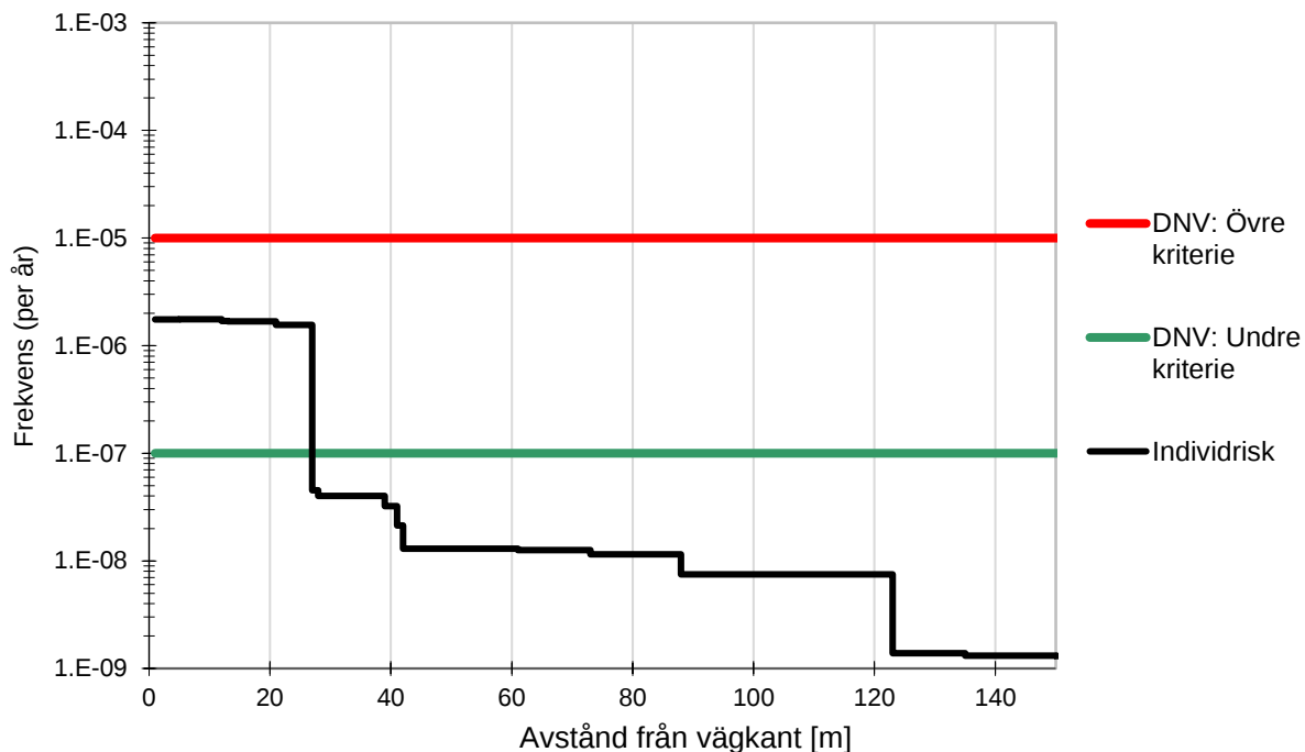
Figur 10. Individrisknivå med avseende på farligt gods-transporter på väg 268
