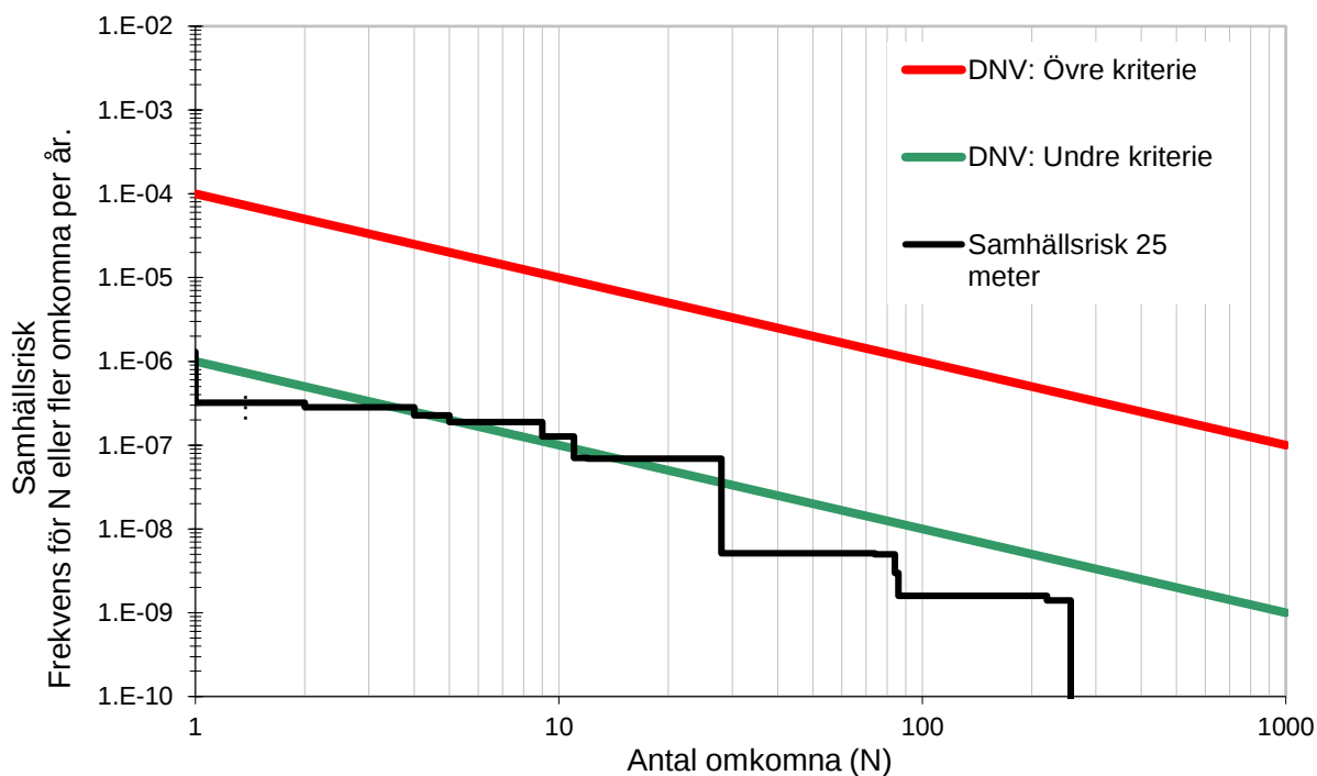
Figur 11. Samhällsrisknivå med avseende på farligt gods-transporter på väg 268
